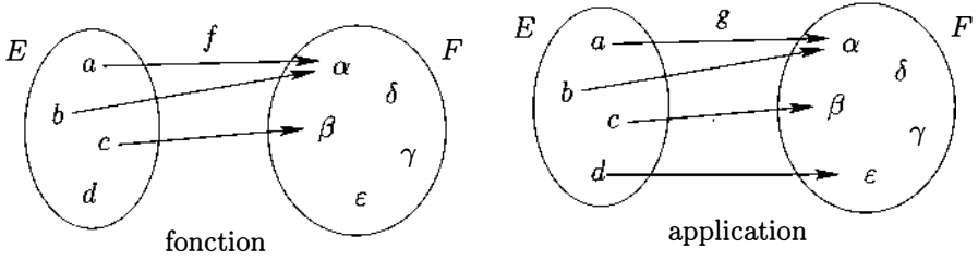
Fig. 7 Diagrammes sagittaux représentant une fonction f : E \longrightarrow F (dessin de gauche) et une application g : E \longrightarrow F (dessin de droite) avec E = \{a, b, c, d\} et F = \{\alpha, \beta, \gamma, \delta, \varepsilon\} .
