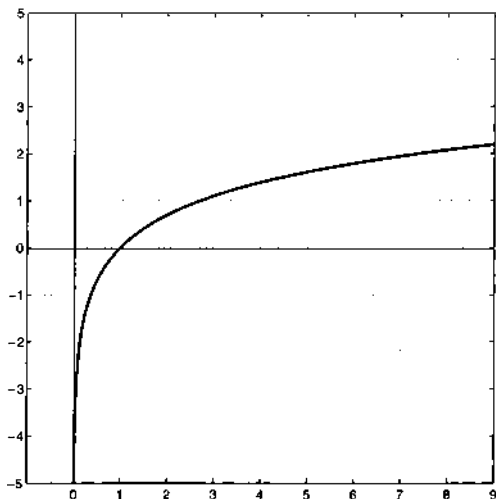
Fig. 4 Représentation graphique de la fonction logarithme népérien.
