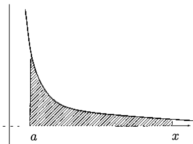
Fig. 1 \int_a^x f(t) dt représente l'aire algébrique hachurée.
