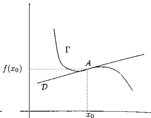
Fig. 12 Cas \nu impair et f^{(\nu)}(x_0) < 0 .
