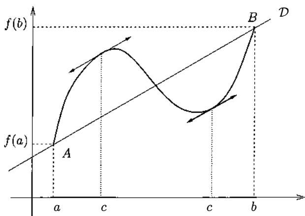
Fig. 5 Interprétation graphique du théorème des accroissements finis.
