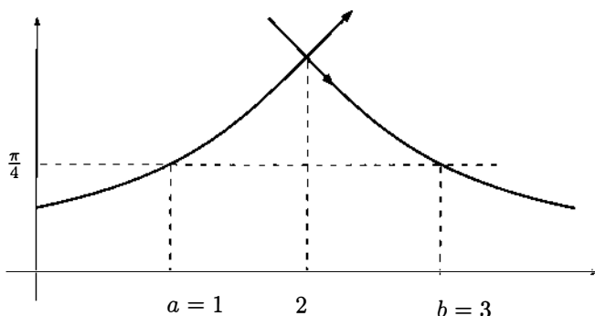
Fig. 4 Représentation graphique de f : x \mapsto \left| \arctan\left(\frac{1}{x-2}\right) \right| .
